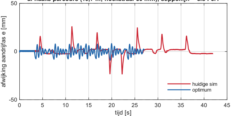
a. haaks parcours (10,7 m, hoekstraal 30 mm); stippellijn = eis F3.1
